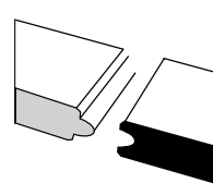
incastro maschio / femmina sulle teste
